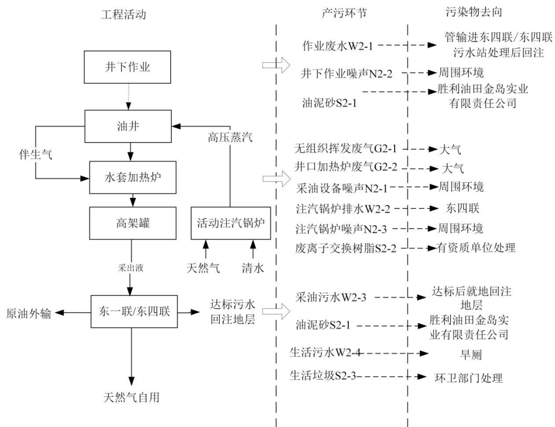
图 3-3 运营期工艺流程及产污环节图
