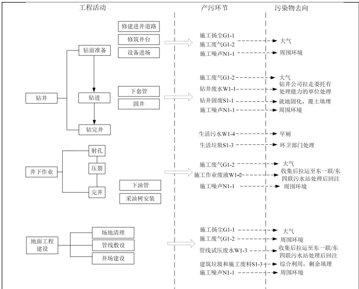
图 3-2 施工期工艺流程及产污环节图
