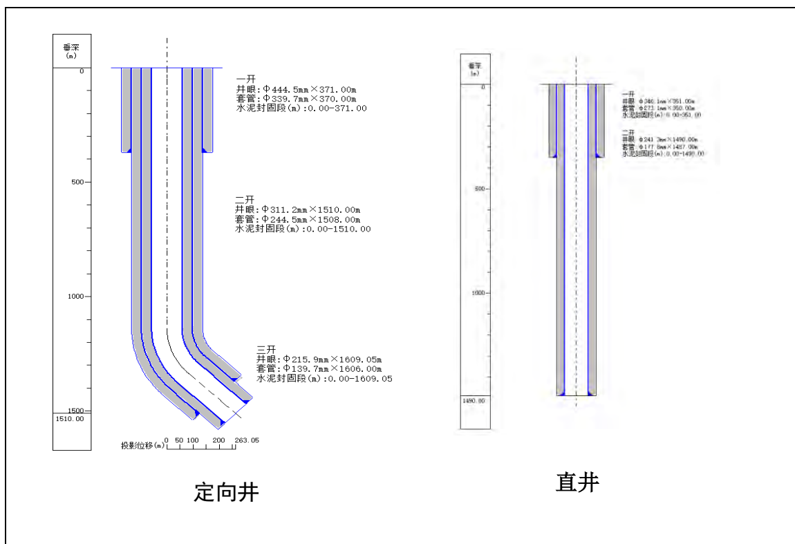
图 3-1 井身结构示意图
